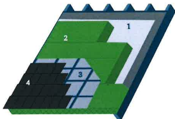
1. Dampscherem | 2. Isolatie | 3. Onderdak | 4. Dakbekleding
