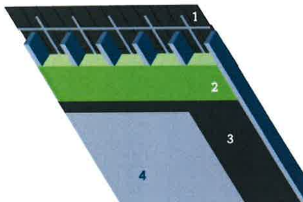
1. Onderdak | 2. Isolatie | 3. Dampscherem | 4. binnenafwerking
