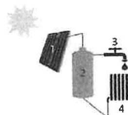
1 Zonnecollector | 2 Opslagvat zonnecollector 3 Sanitair warm water 4 Afgeleide warmte ruimteverwarming (oprecht)
