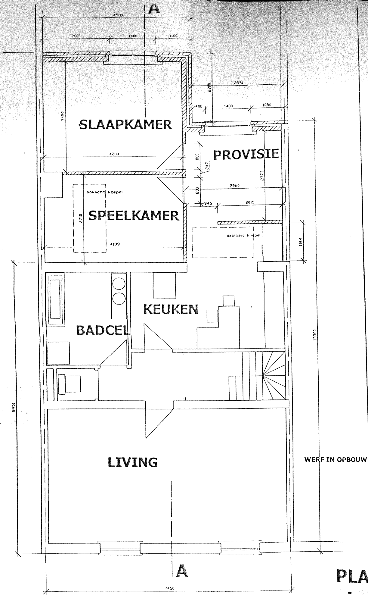
PLAN NIVO 2 nieuwe toestand
