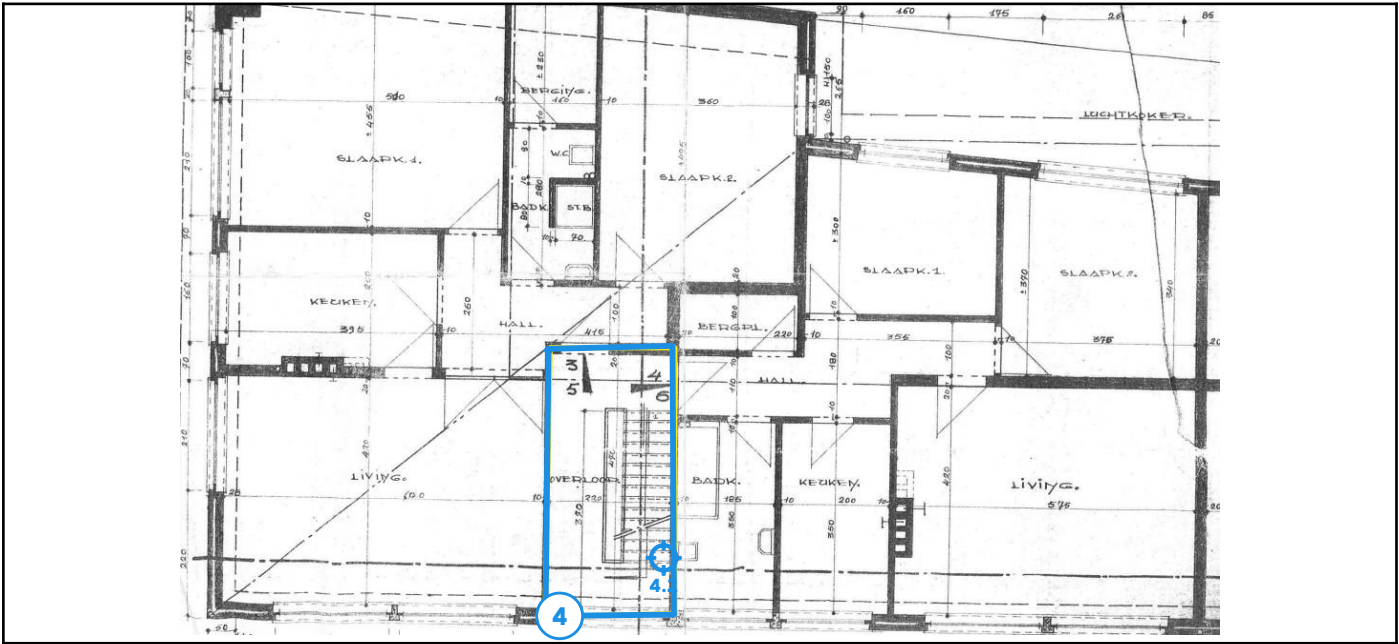
Legende van plan 1.7: Hoofdgebouw plan V+2 Pleisterwerk muren
