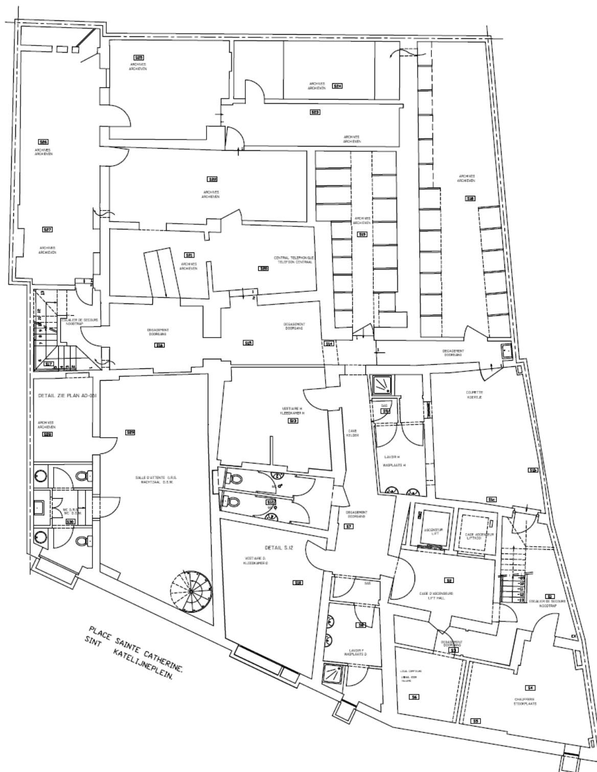
PLAN DU SOUS-SOL. PLAN VAN KELDERVERDIEPING.
