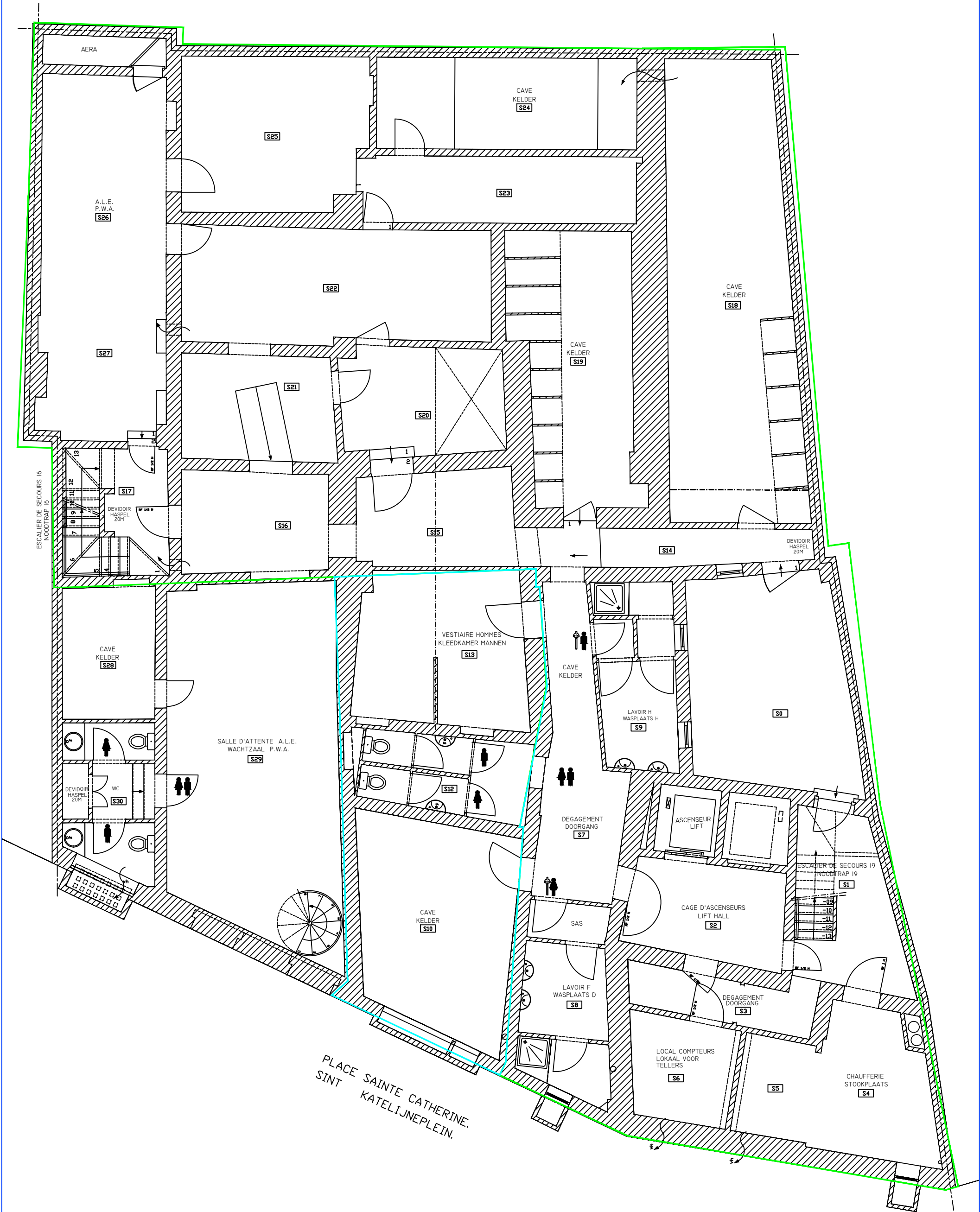
PLAN DU SOUS-SOL. PLAN VAN KELDERVERDIEPING.
