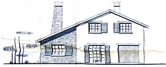
FACADE EST.
