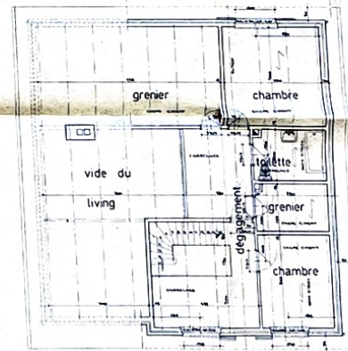
ETAGE
