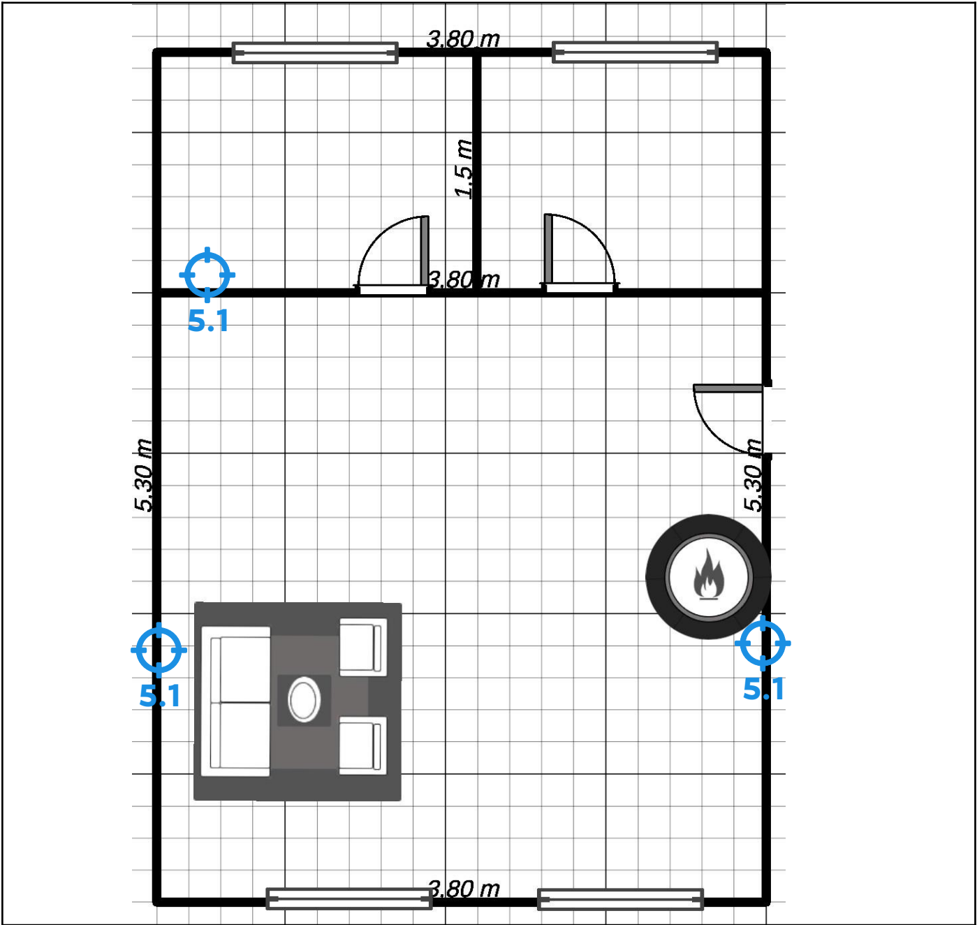
Legende van plan 1.2: Verdieping 1
