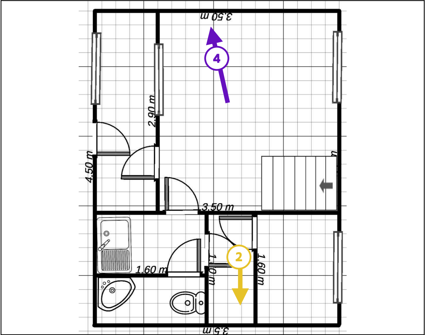
Legende van plan 1.2: Gelijkvloers 1.1
