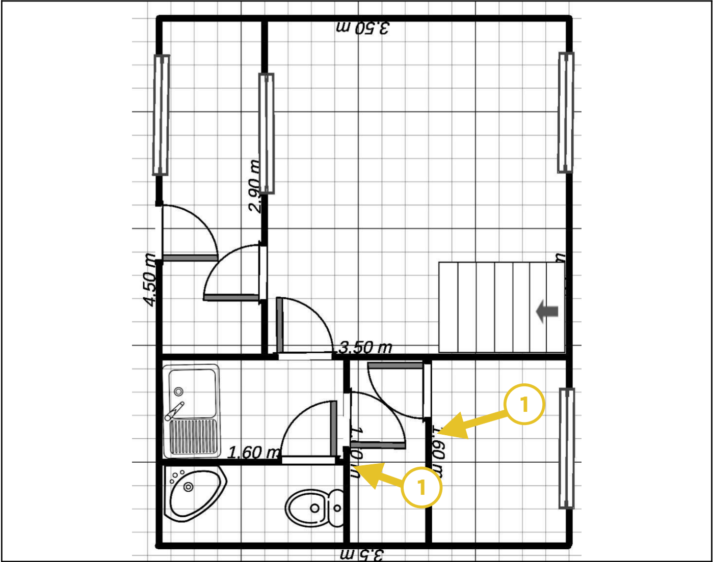
Legende van plan 1.3: Gelijkvloers 1.2
