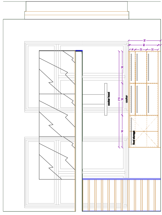
RIGHT ELEVATION
