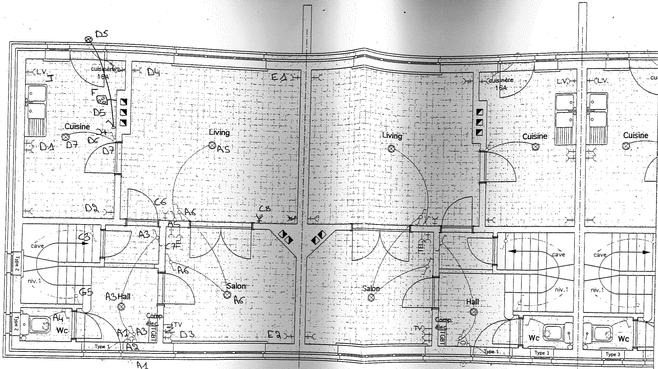
Vue en plan Rez-de-chaussée - partie gauche
