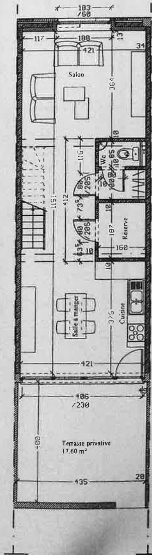
Rez-de-chaussée
