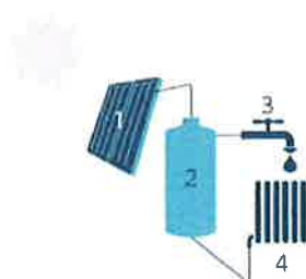
1 Zonnecollector 2 Opslagvat voor warm water 3 Sanitair warm water 4 Ruimteverwarming
