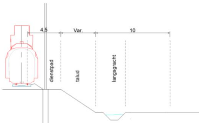
Schematische voorstelling van de bouwvrije strook met talud
