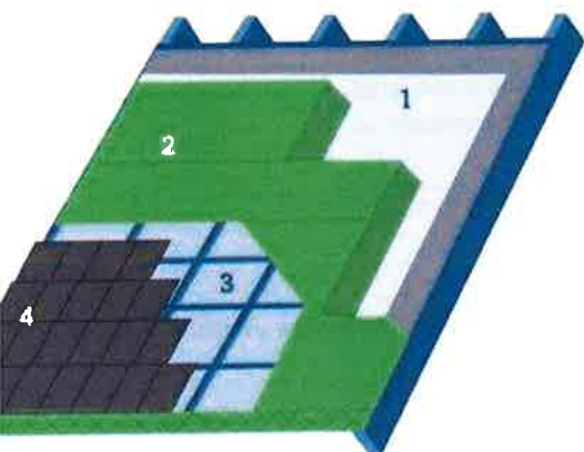
1. Onderdak | 2. Isolatie | 3. Onderdak | 4. Dakbekleding
