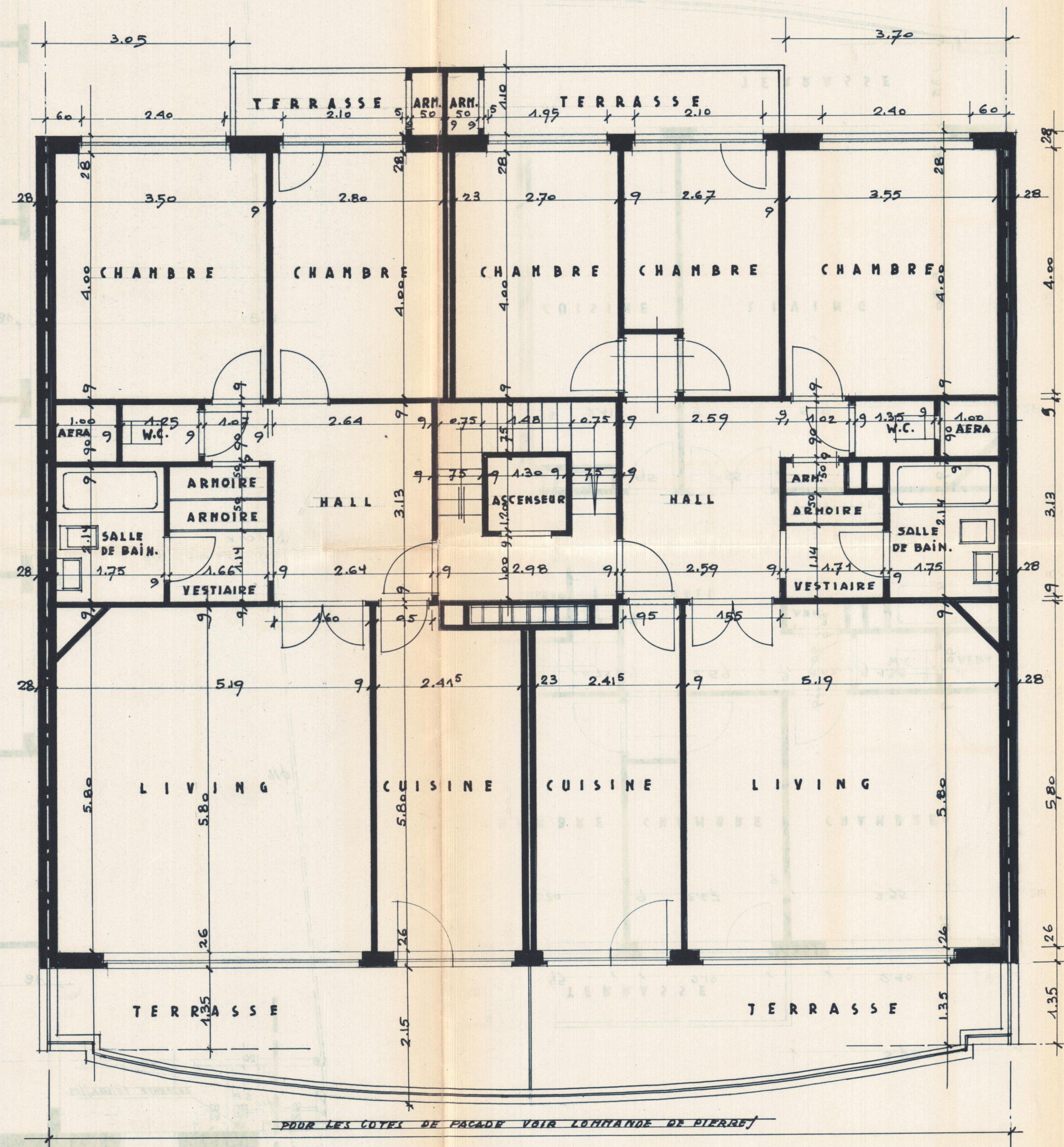
PLAN DE L'ETAGE EN RECU.
