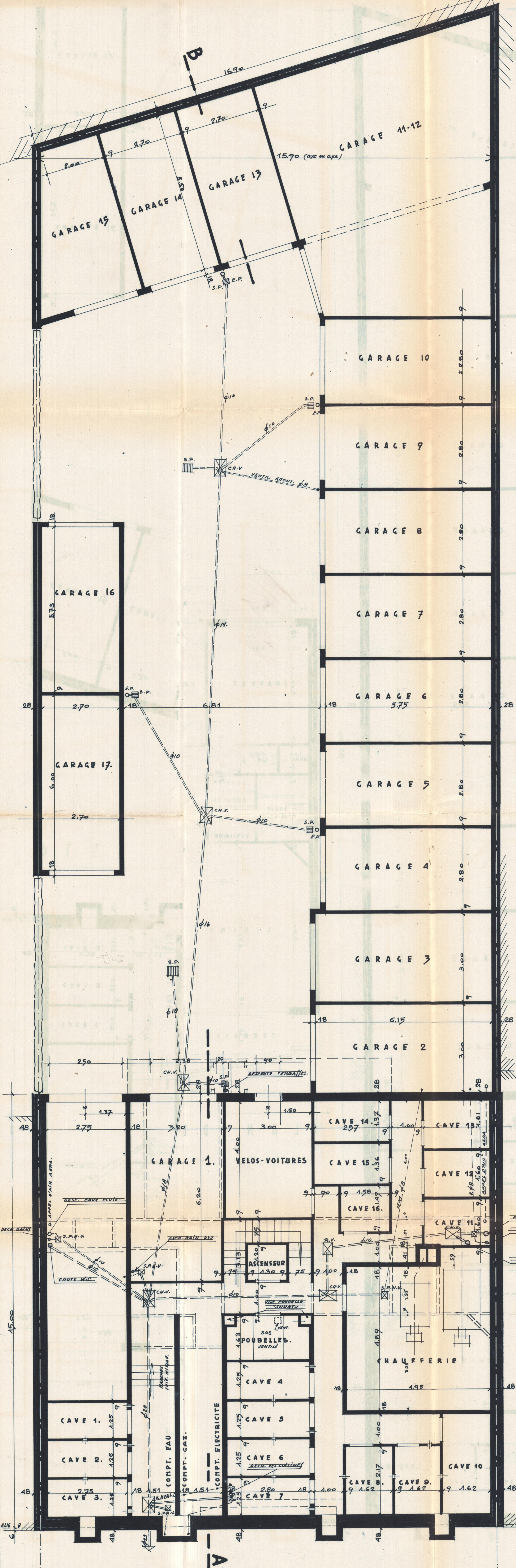
PLAN DES SOUS-SOLS.
