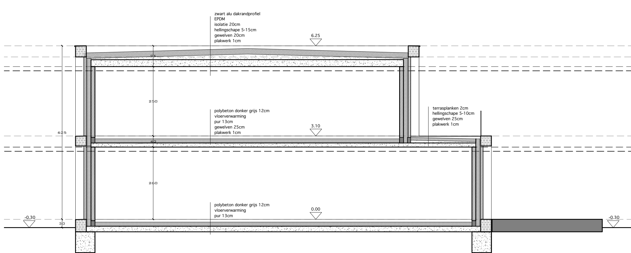
SNEDE
