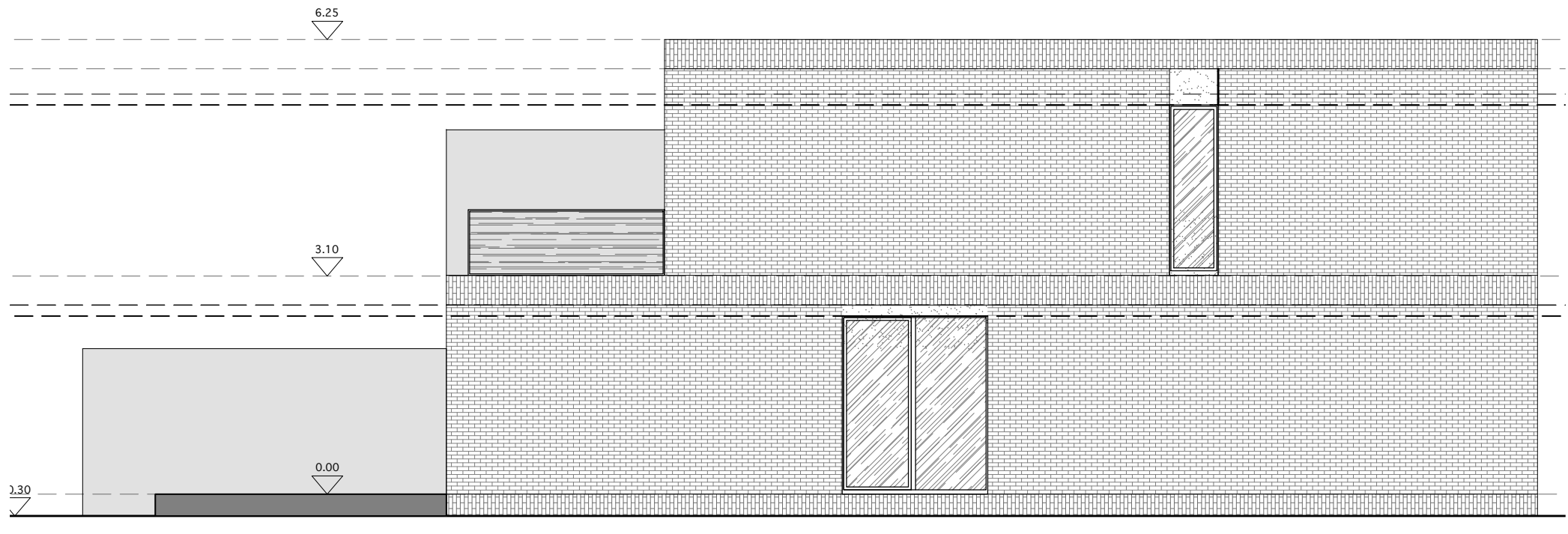
ZIJGEVEL
