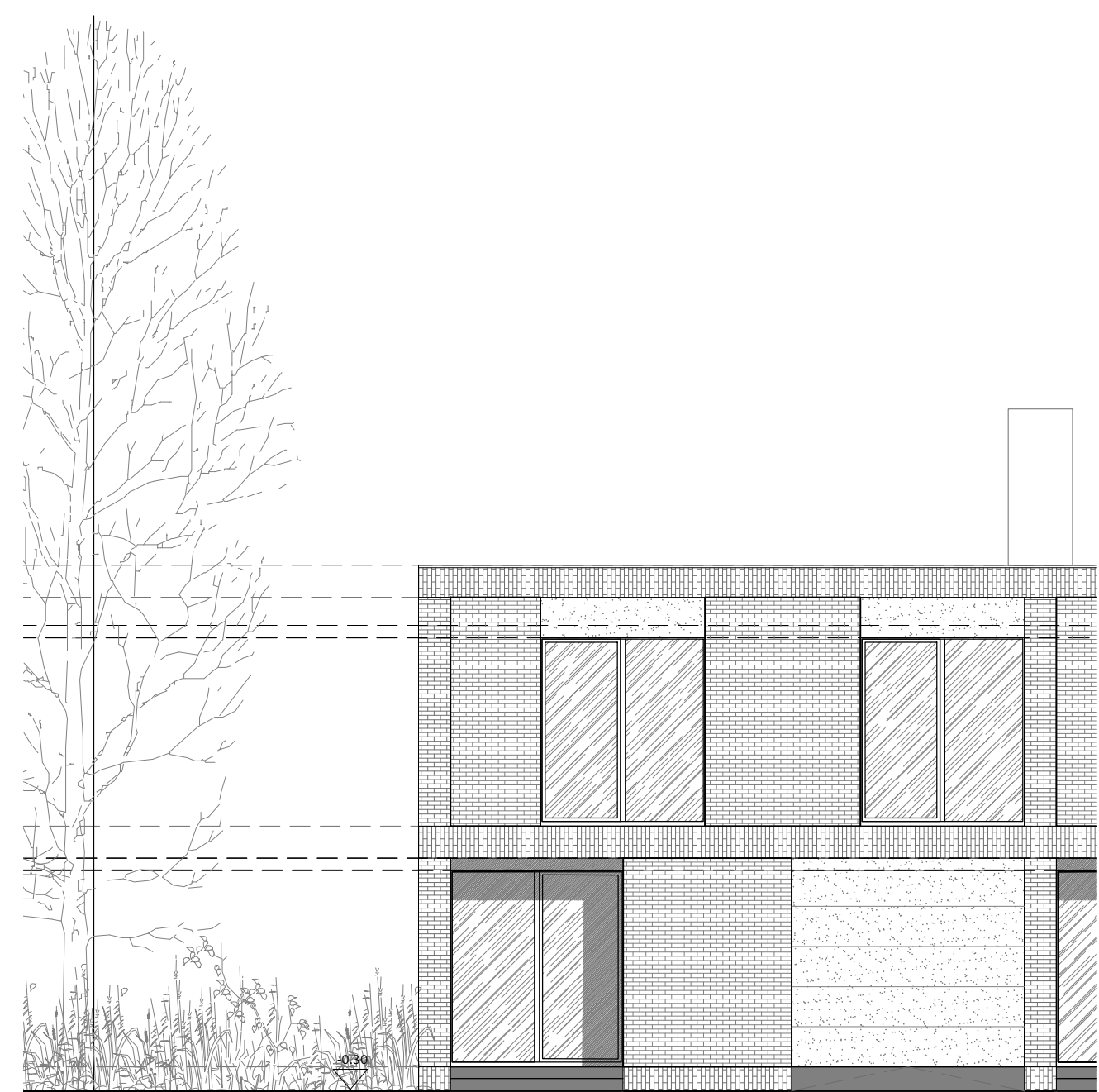
ACHTERGEVEL
