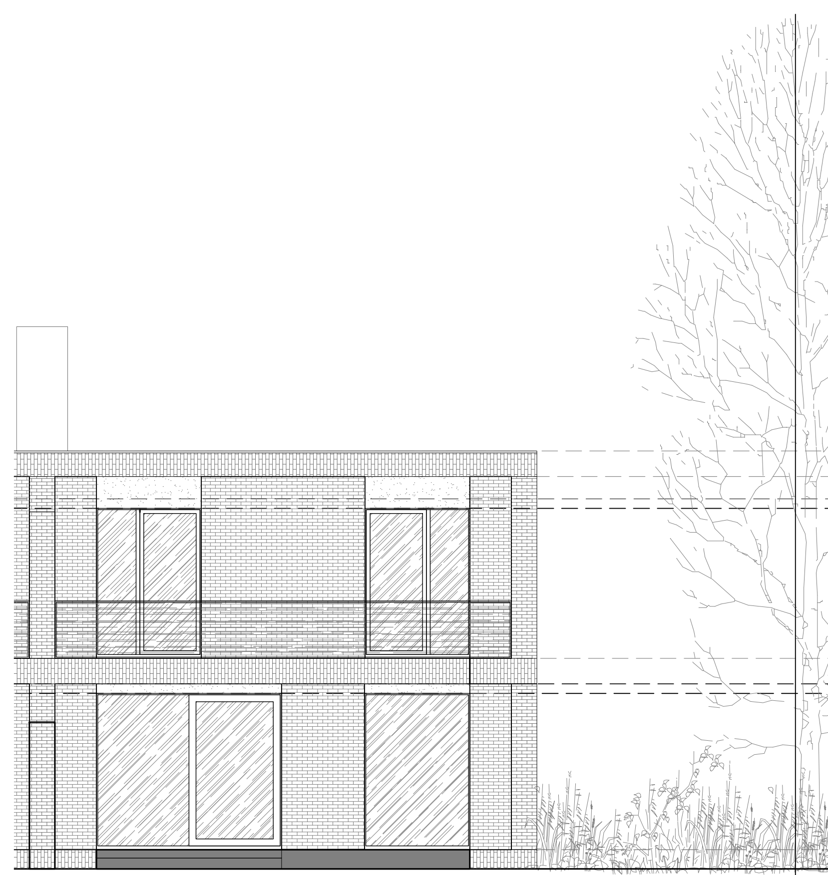
ACHTERGEVEL
