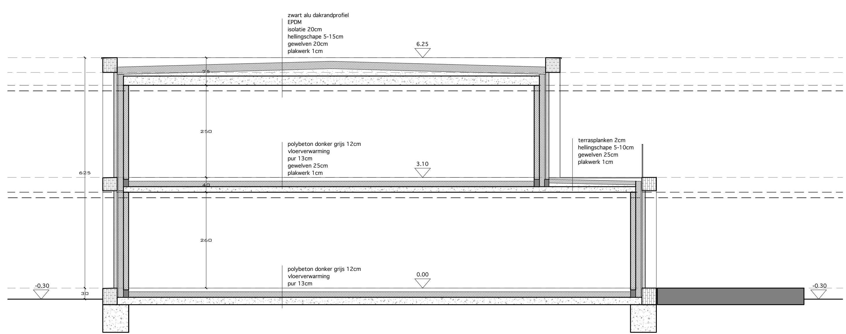
SNEDE
