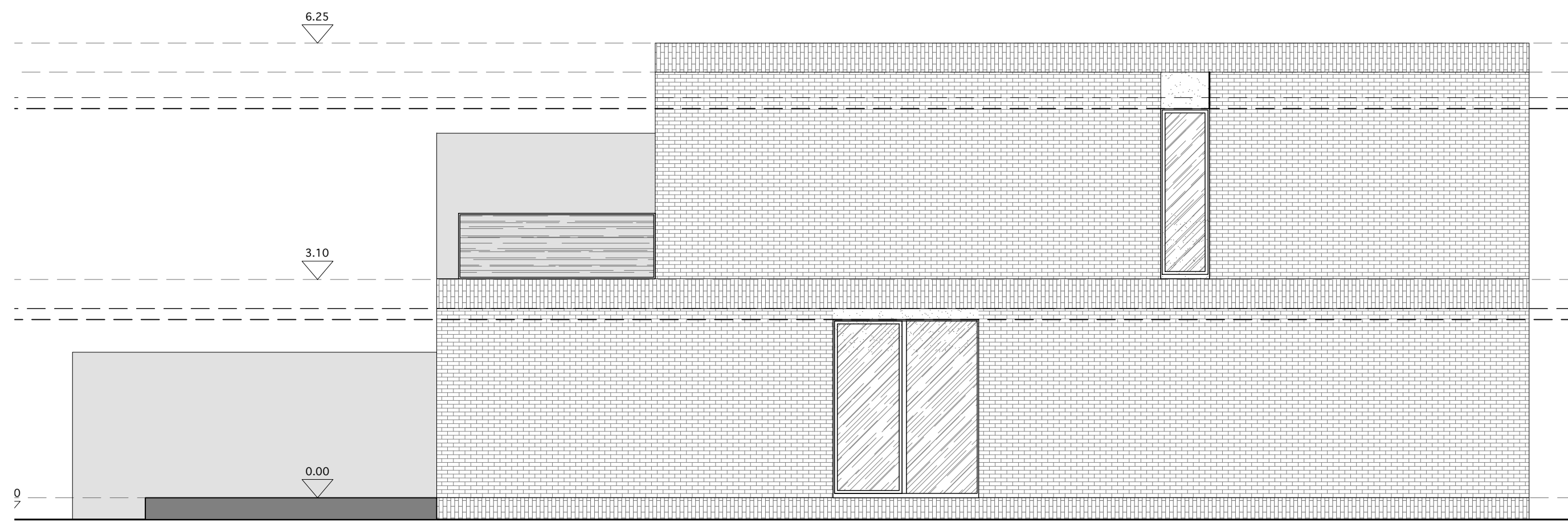
ZIJGEVEL
