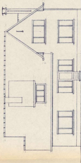
ACHTERGEVEL
