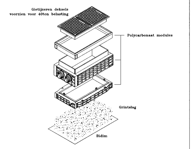
PLAATSIING VAN EEN POLYCARBONAAT MODULAIRE LASKAMER TYPE EK388
