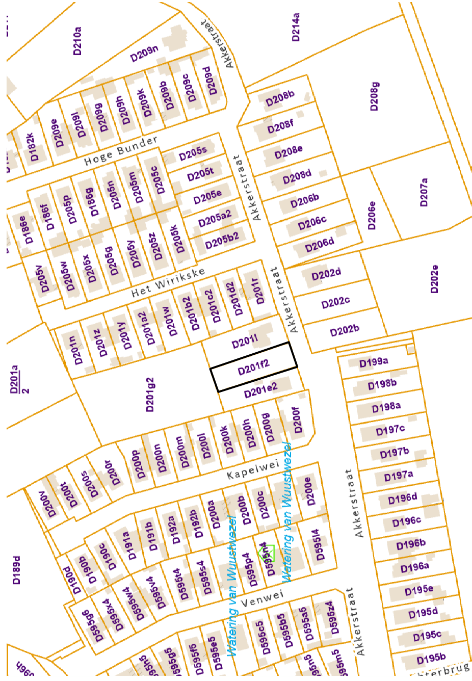
LIGGINGSPLAN: ±1/2500
