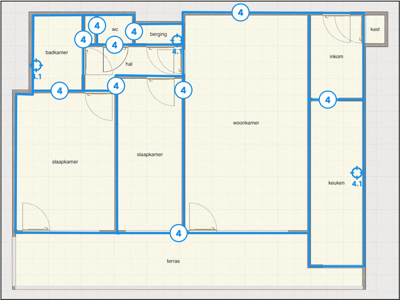
Legende van plan 1.2: Appartement pleisterwerk binnenwanden
