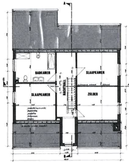
VERDIEPINGSPLAN
