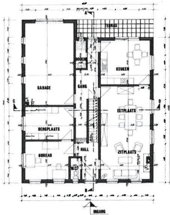
GRONDPLAN
