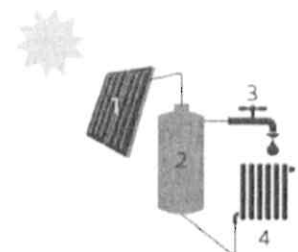
1. Zonnecollector 2. Opslagvat zonnecollector 3. Sanitair warm water afnemer 4. Radiator * Het rendement van zonnecollectoren is lager in de winter dan in de zomer.
