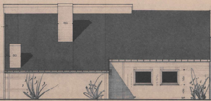
ZUGEVEL LINKS
