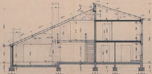
DOORSNEDE A.A.
