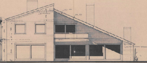
ACHTERGEVEL
