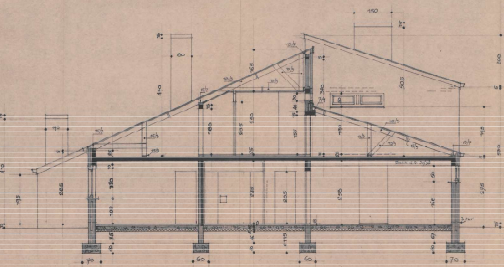
DOORSNEDE D.D.
