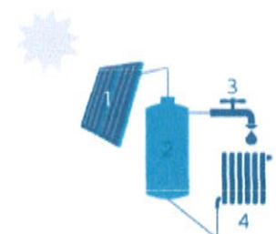
1 Zonnecollector | 2 Opslagvat | 3 Sanitair warm water of ruimteverwarming voor zonnecollector | 4 Radiator
