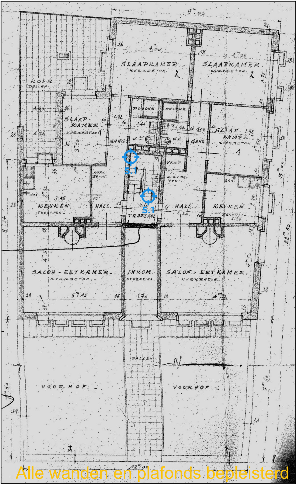
Legende van plan 1.2: Gelijkvloers GD
