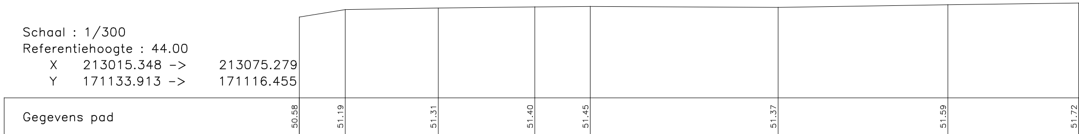
LENGTEPROFIEL A - B
