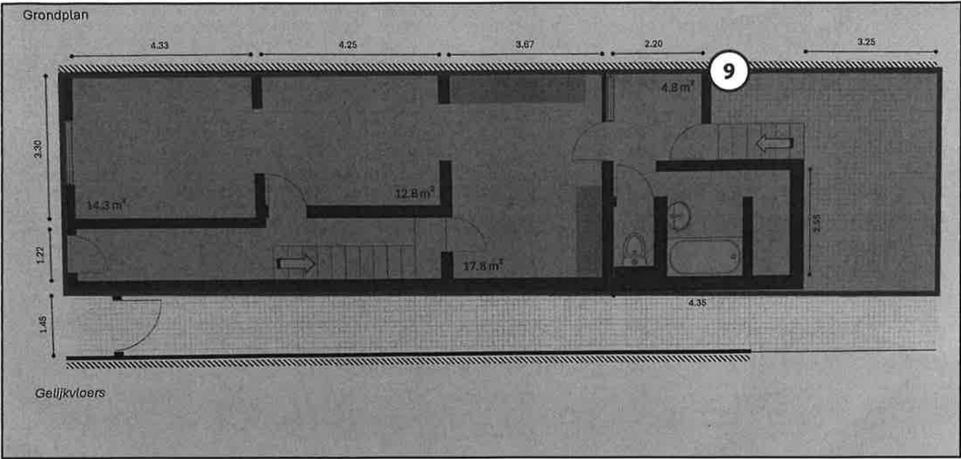
Legende van plan 1.4: Plan gelijkvloers
