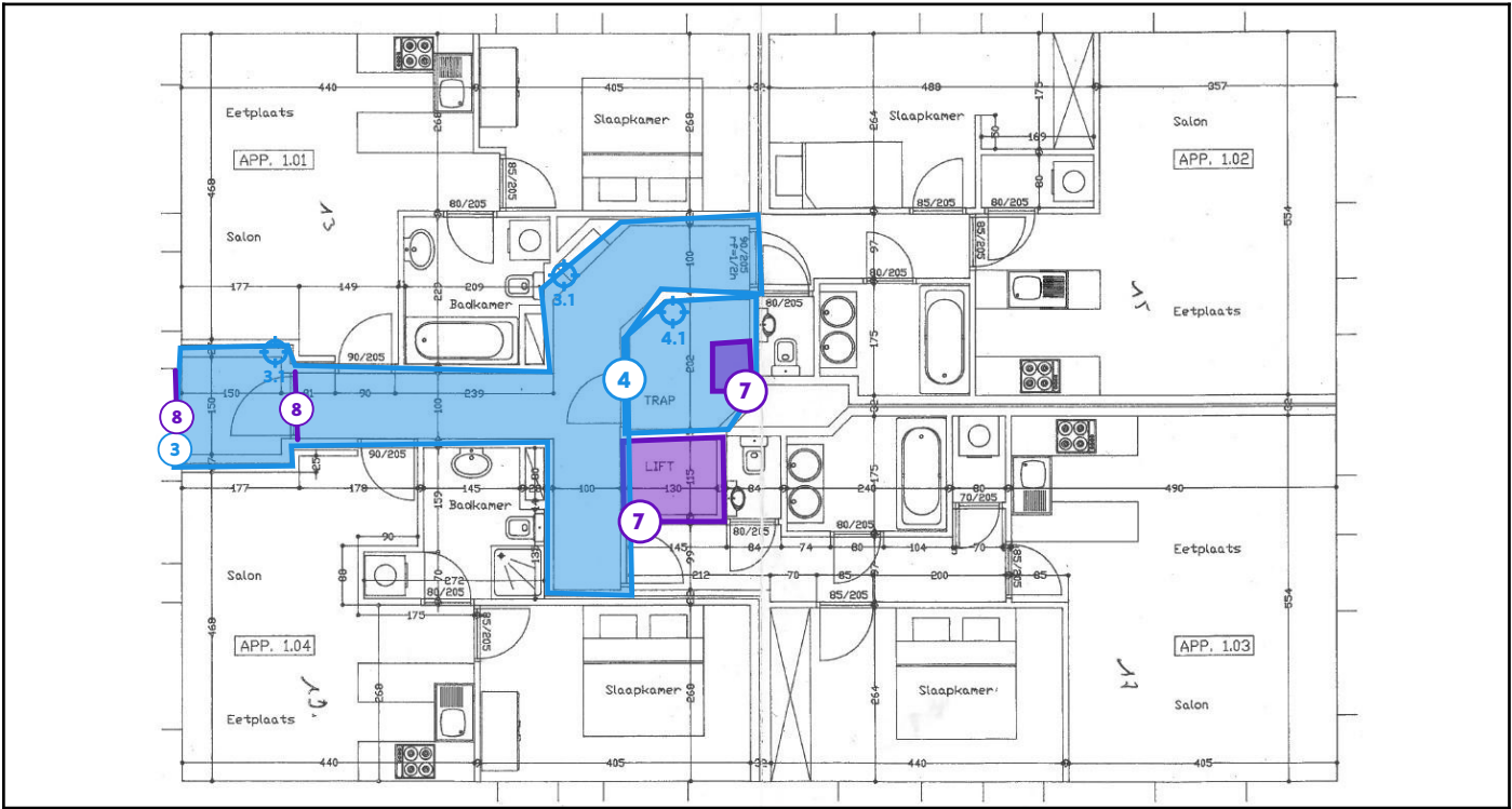
Legende van plan 2.1: GLV
