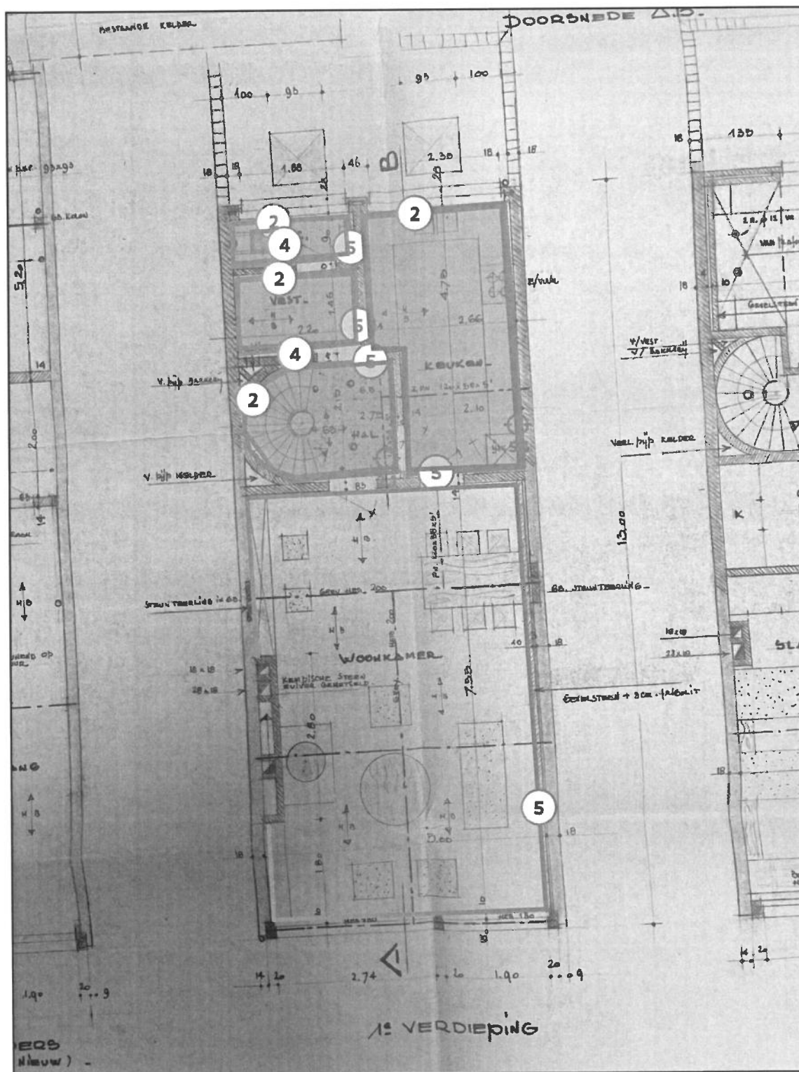
Legende van plan 1.6: Situatieplan 1ste verdiep voorbouw
