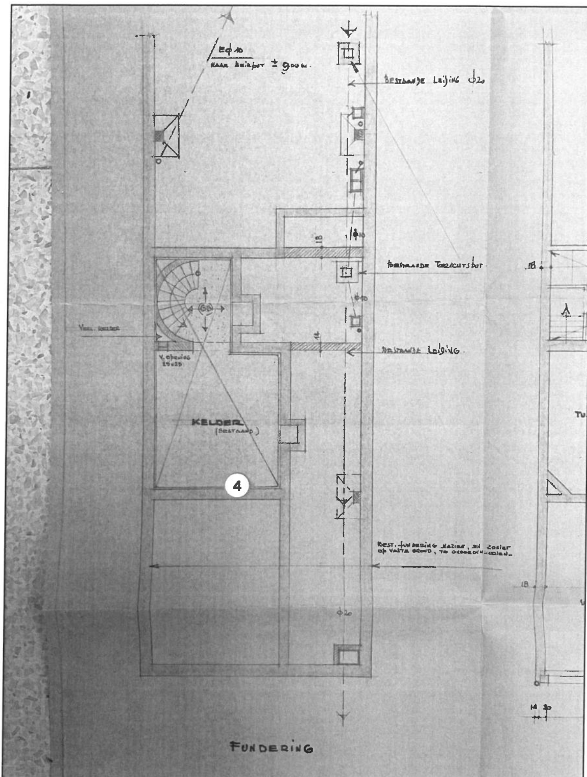
Legende van plan 1.2: Situatieplan fundering voorbouw
