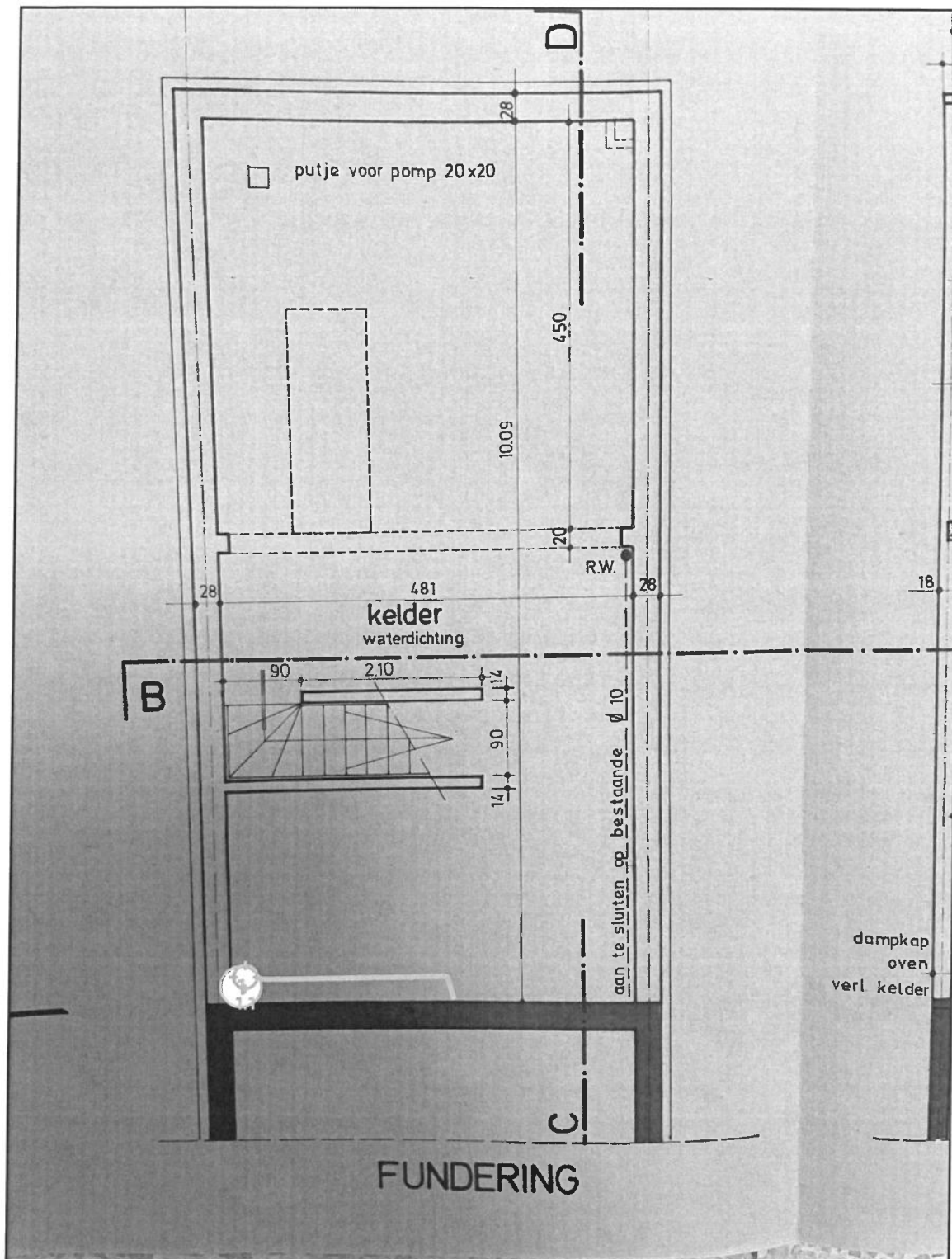
Legende van plan 1.3: Situatieplan fundering achterbouw
