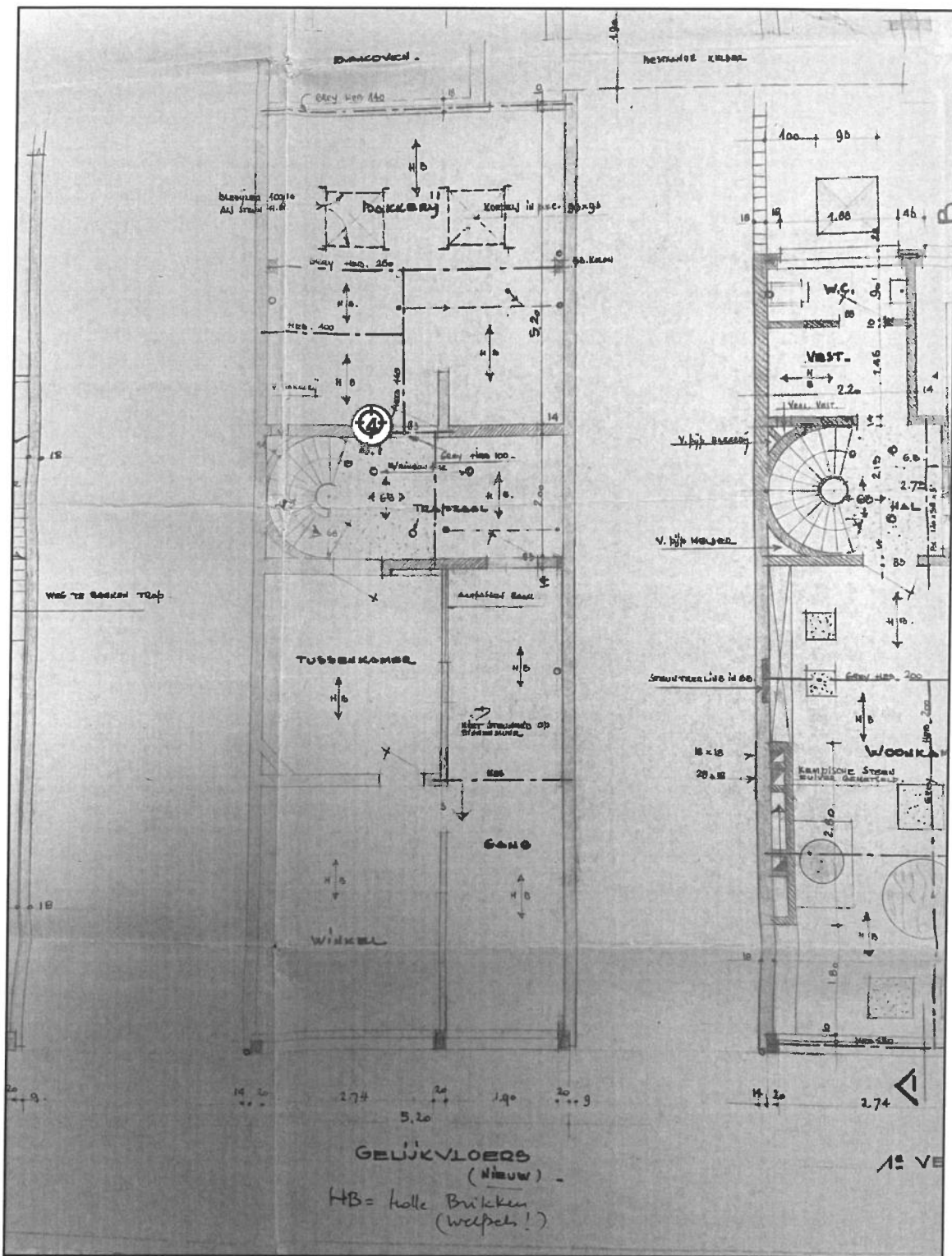
Legende van plan 1.4: Situatieplan gelijkvloers voorbouw
