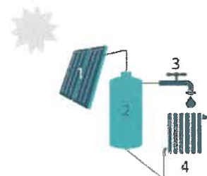
1 Zonnecollector | 2 Opslagvat voor warm water | 3 Sanitair warm water | 4 Radiatoren voor ruimteverwarming
