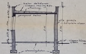
doorsnede : a.b.
