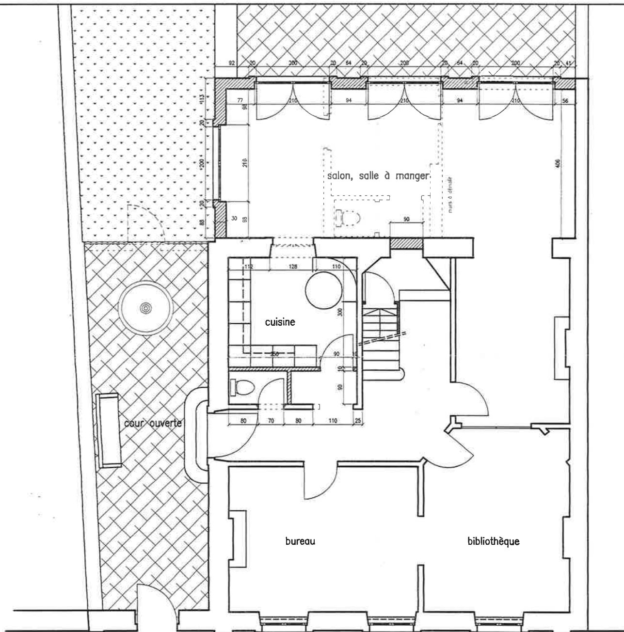
rez de chaussée projeté
