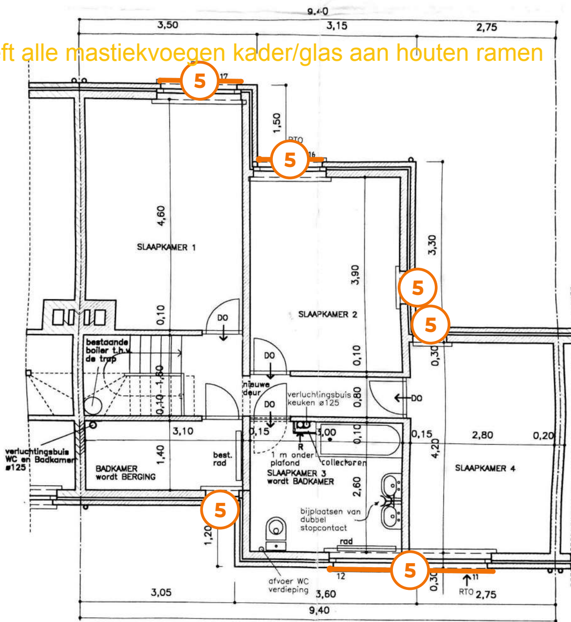
PLAN VERDIEPING Type 1 : slaapkamer 3 wordt badkamer
