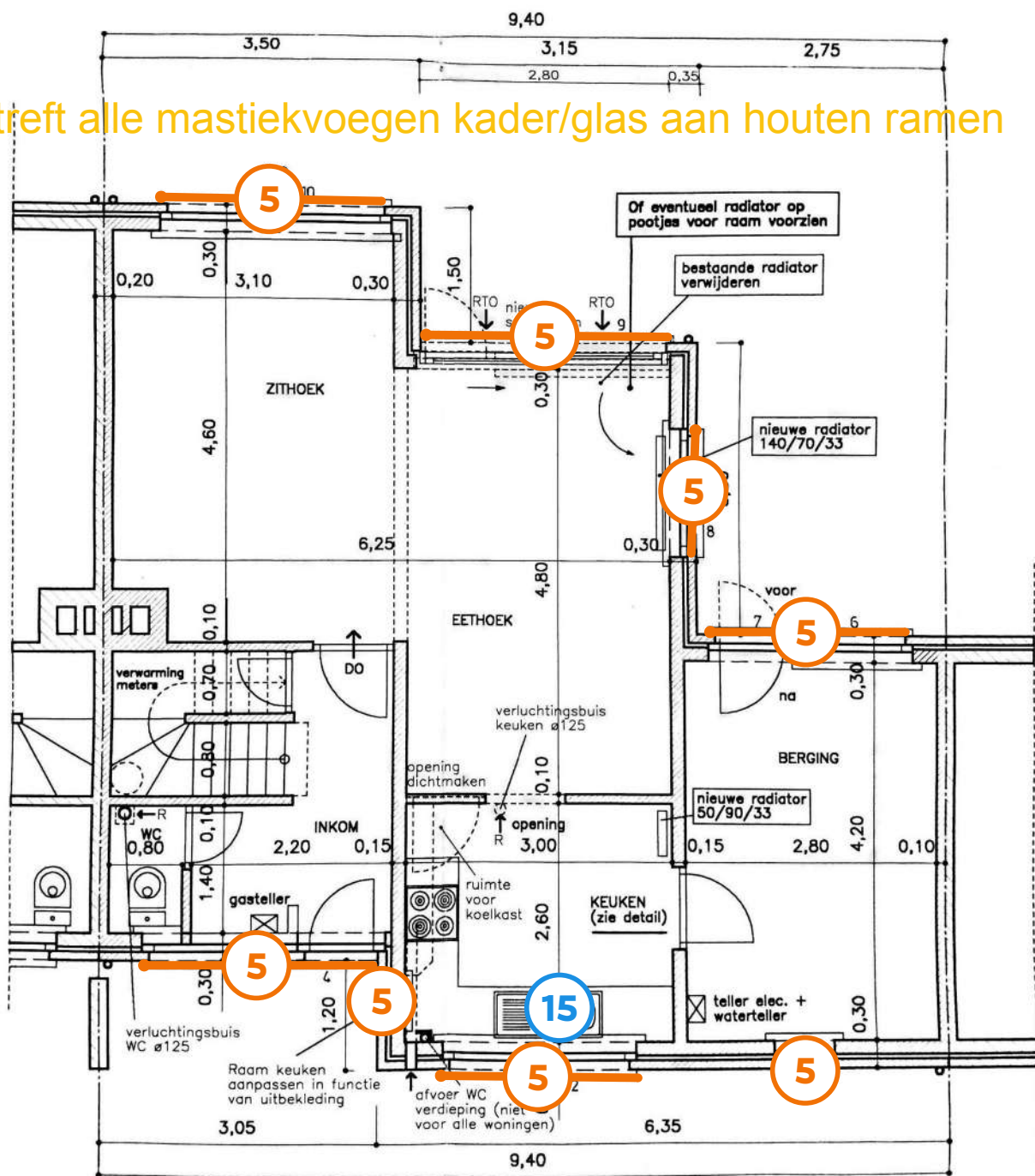
PLAN GELIJKVLOERS Type 1
