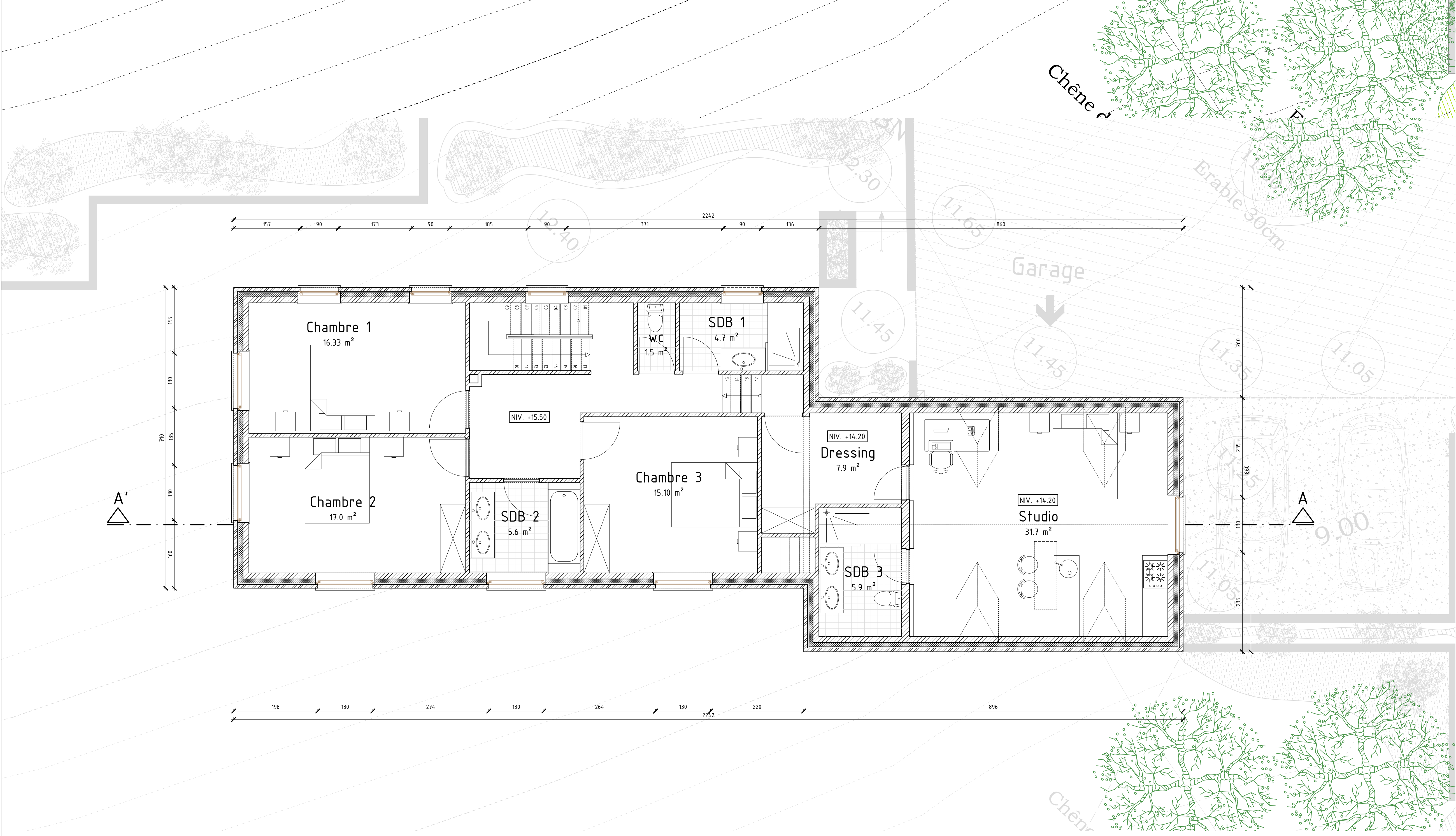
Plan Etage
