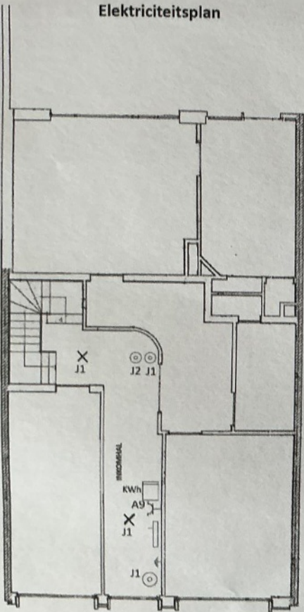
Gelijkvloers
