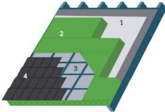
1. Dampscherm | 2. Isolatatie | 3. Onderdak | 4. Dakbedekking
