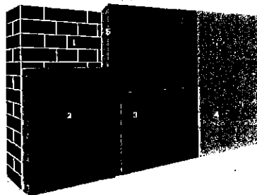
1. Bultengevel | 2. Isolatie | 3. Dampscherm | 4. Binnenafwerking | 5. Stijl- en regelwerk (optioneel)
