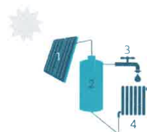
(1) Zonnecollector (2) Opslagvat zonneboiler (3) Sanitair water (4) Warmtebron voor ruimteverwarming of verwarming
