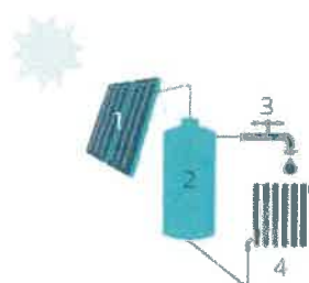
1 Zonnecollector | 2 Opslagvat zonnepomp | 3 Sanitair warm water | 4 Afgiftelid element voor ruimteverwarming (optioneel)
