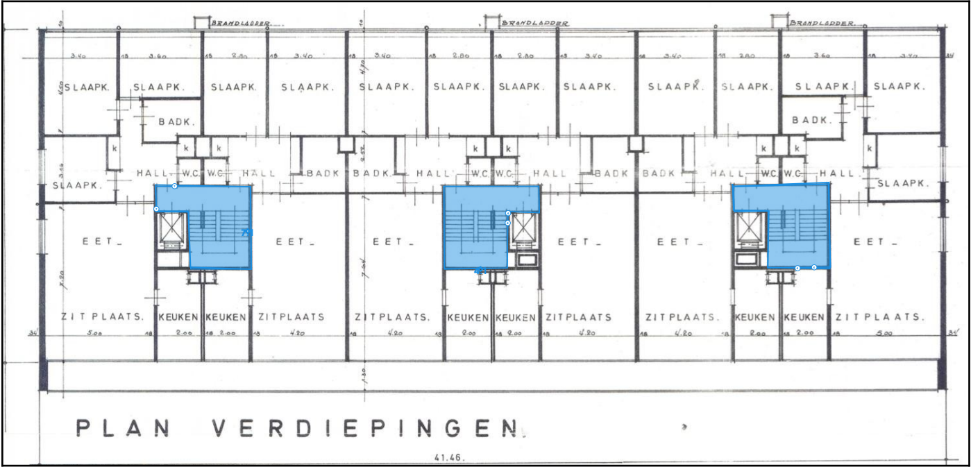
Legende van plan 1.5: Verdieping +3
