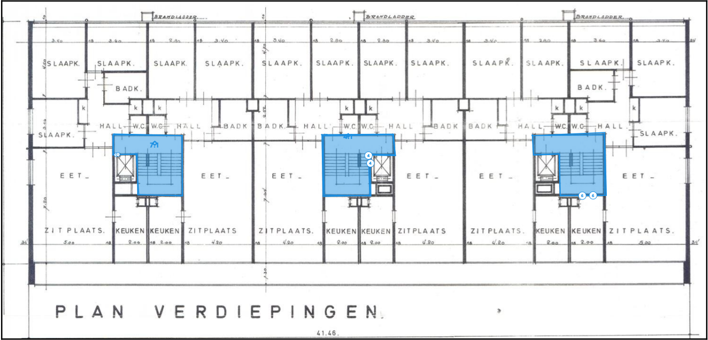
Legende van plan 1.9: Verdieping +7
