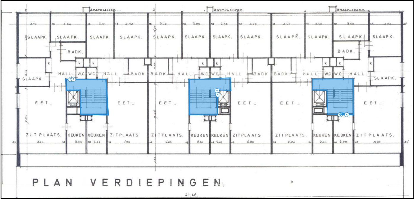
Legende van plan 1.4: Verdieping +2
