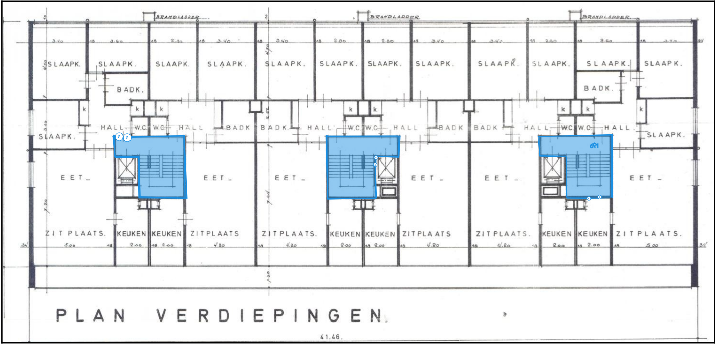
Legende van plan 1.10: Verdieping +8
