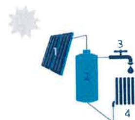
1 Zonnecollector | 2 Opslagvat zonnecollector | 3 Sanitair warm water (koud) 4 Radiator voor ruimteverwarming (koudwater)
