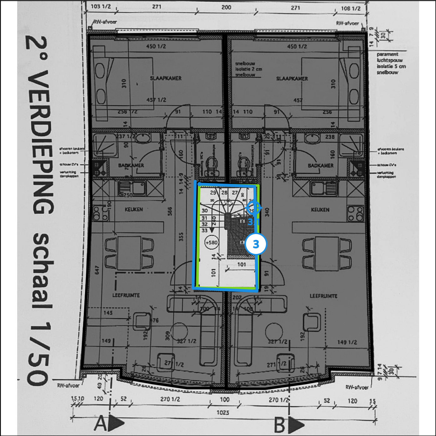
Legende van plan 1.4: Grondplan verdieping 2 muur
