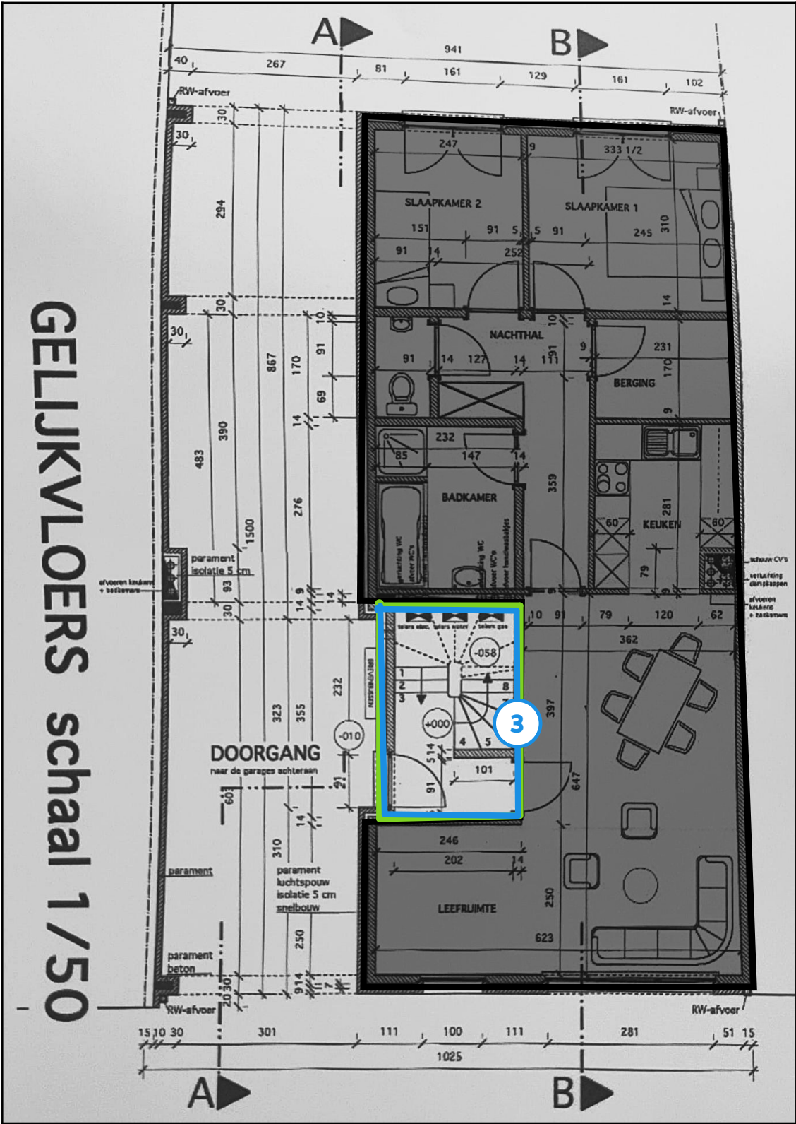
Legende van plan 1.1: Grondplan gelijkvloers muur
