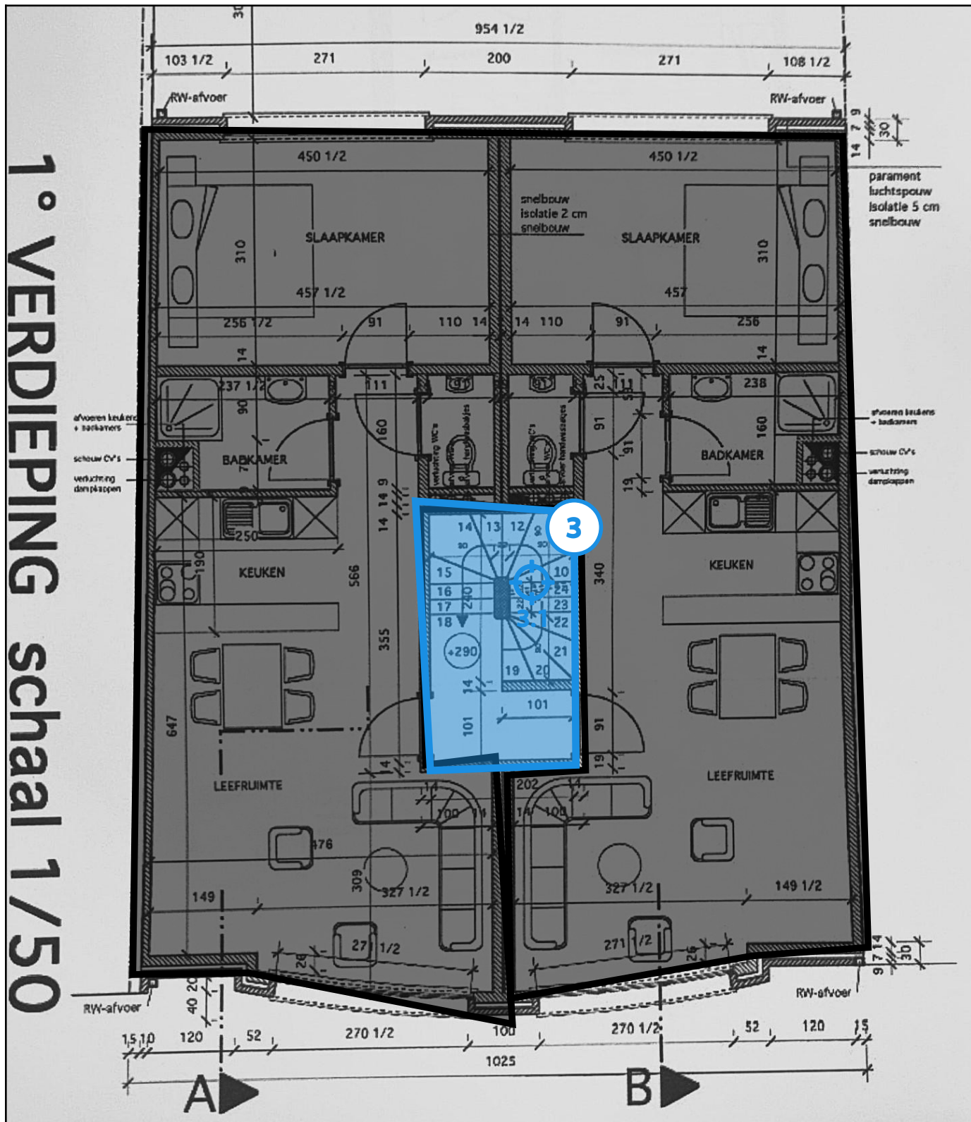
Legende van plan 1.3: Grondplan verdieping 1 plafond
