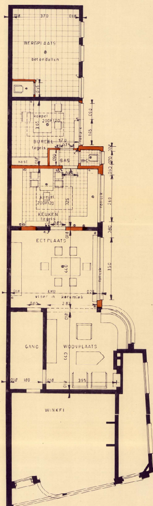
GELIJKVLOERS NIEUW TOESTAND
