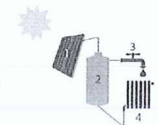
1. Zonnecollector | 2. Opslagvat zonnecollector | 3. Sanitair warm water | 4. Afgifte-element voor ruimteverwarming (optioneel)
