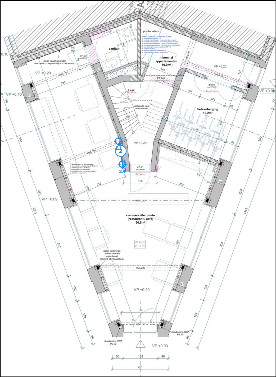
Legende van plan 1.2: Plan gelijkvloers
