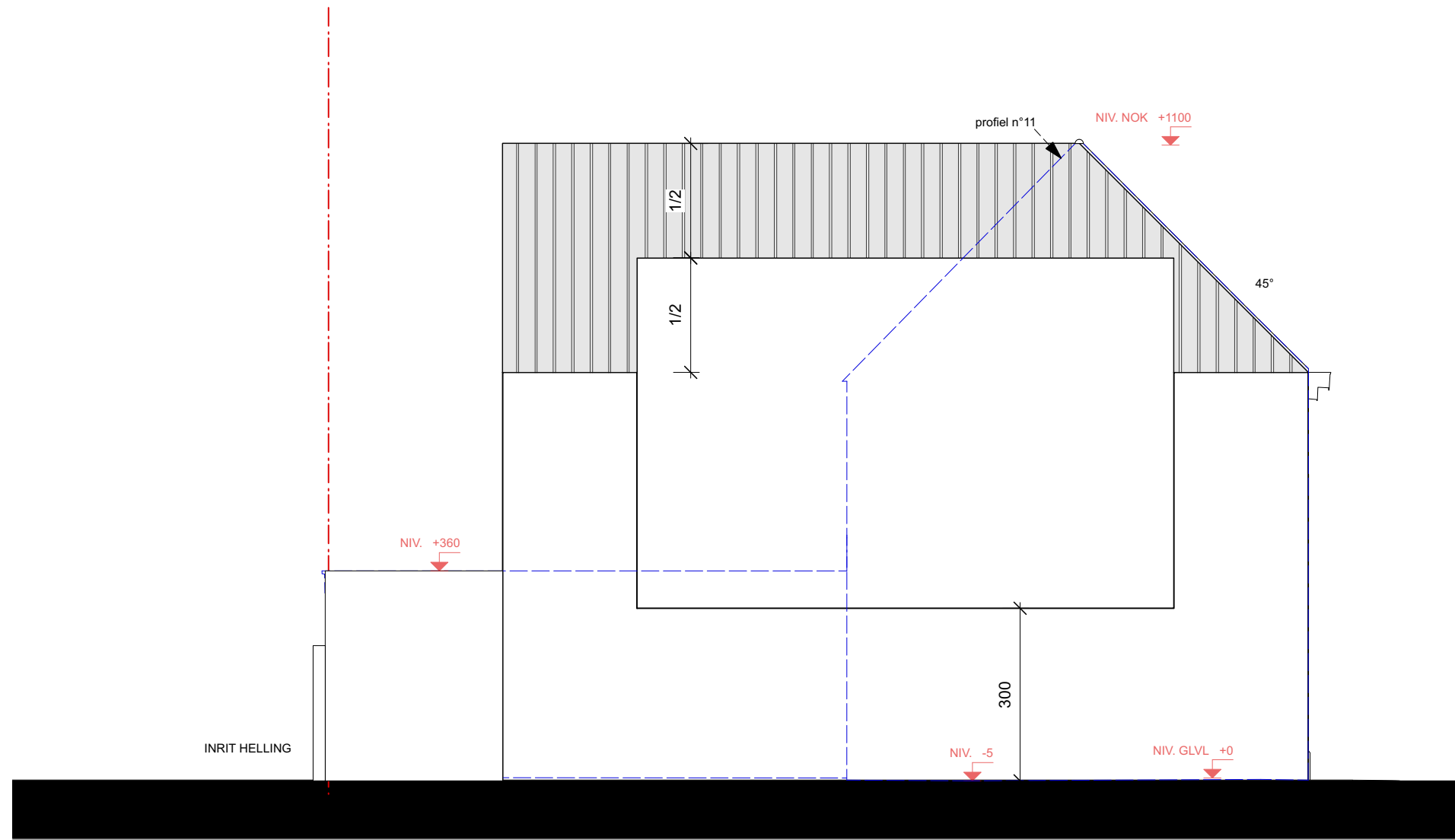
GEVEL SCHOOLSTRAAT SCHAAL: 1:100
