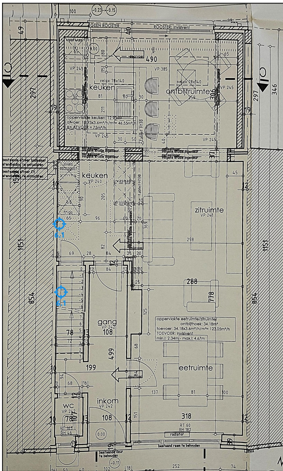
Legende van plan 1.1: Grondplan +0
