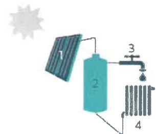
1 Zonnecollector | 2 Opslagvat zonnepanelen 3 Sanitair warm water 4 Radiator-element voor ruimteverwarming
